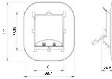
Grundplatte
